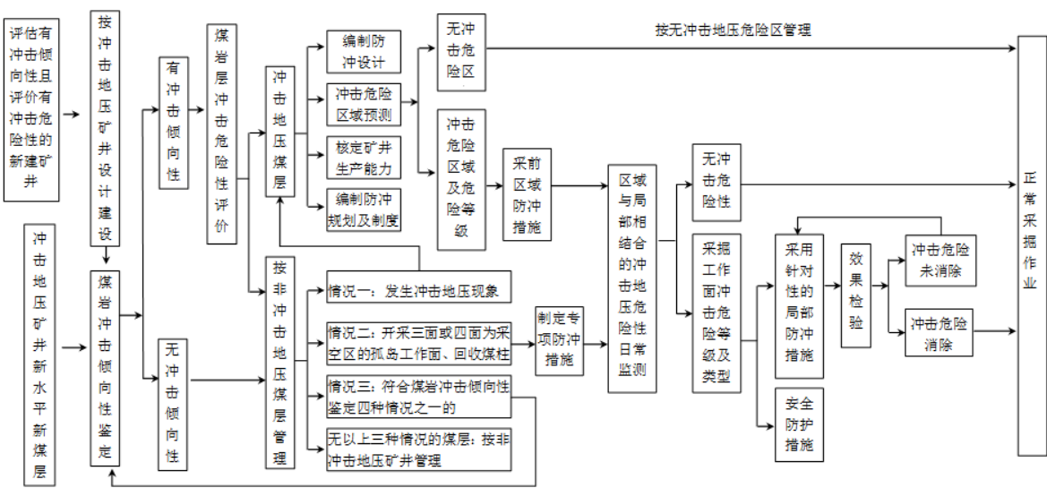
防治煤矿冲击地压基本流程示意图
