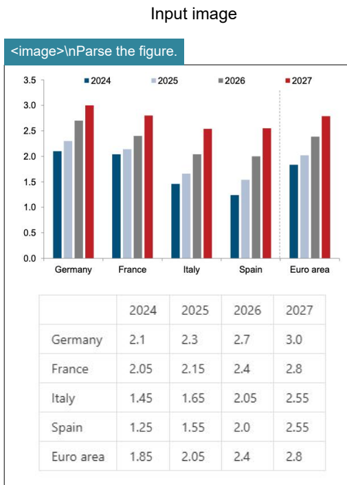
Deep Parsing
