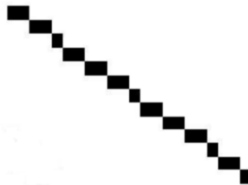
图 4-7 直线走样
