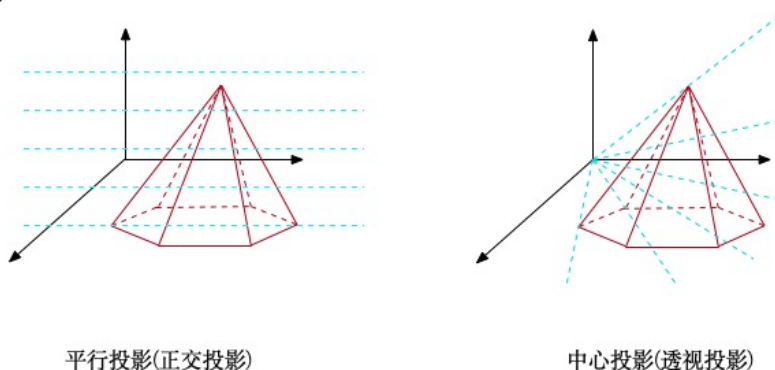
图 3-6 正交投影和透视投影
