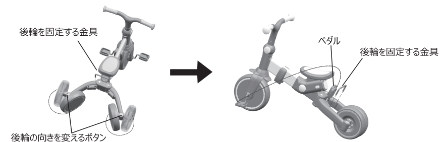
後輪の向きを変えるボタン
